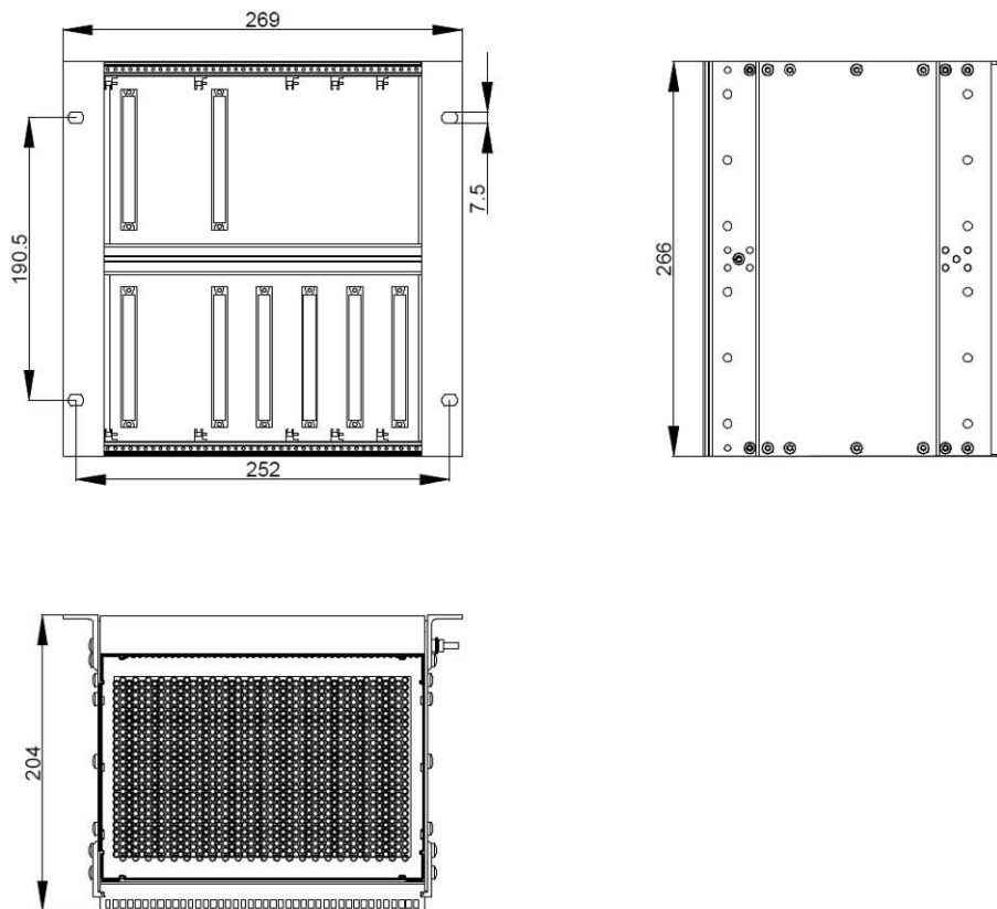
Рисунок 39 - Габаритные размеры крейта на 7 слотов (установка на монтажную панель)
