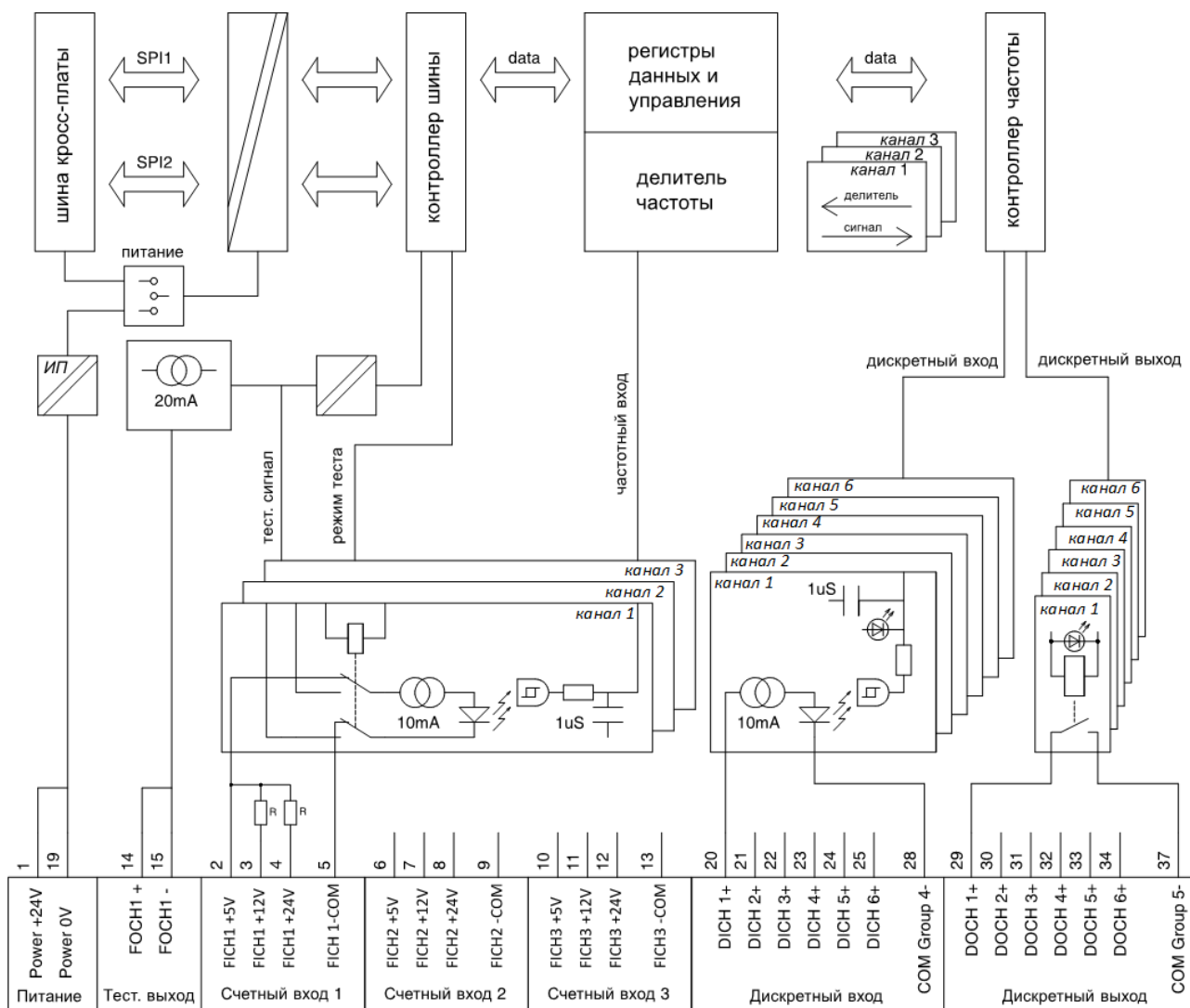
Рисунок 34 - Структурная схема модуля R600 DA 03 011
