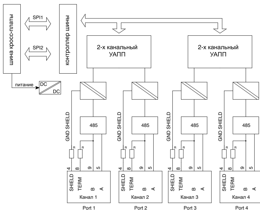
Рисунок 21 - Структурная схема модуля CP 04 011
