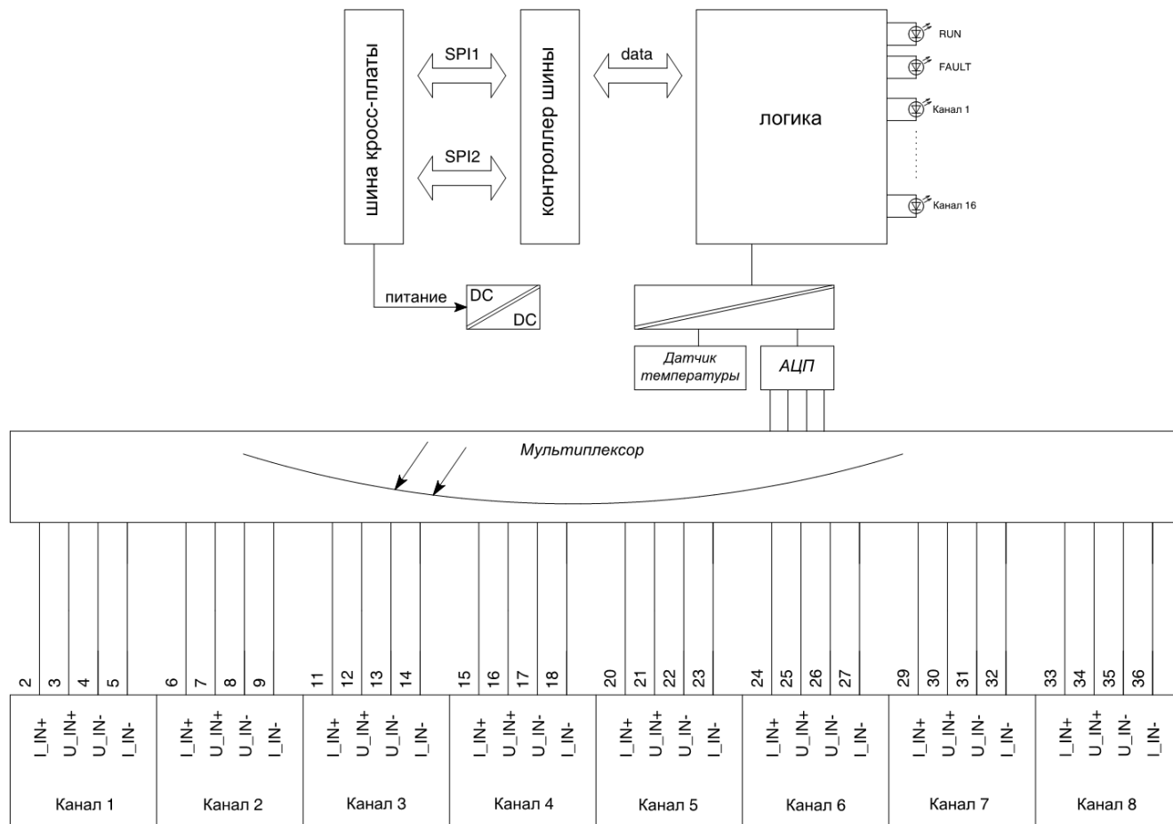
Рисунок 27 - Структурная схема модуля AI 08 031
