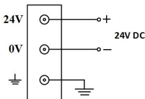
Рисунок 20 - Подключение входного напряжения 24В на модуле PP 14 011
