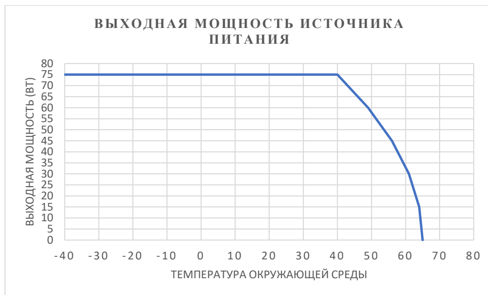
Рисунок 18 – График зависимости мощности источника питания от температуры
