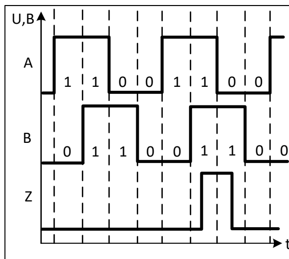
Рисунок 33 – Выходные сигналы энкодера
