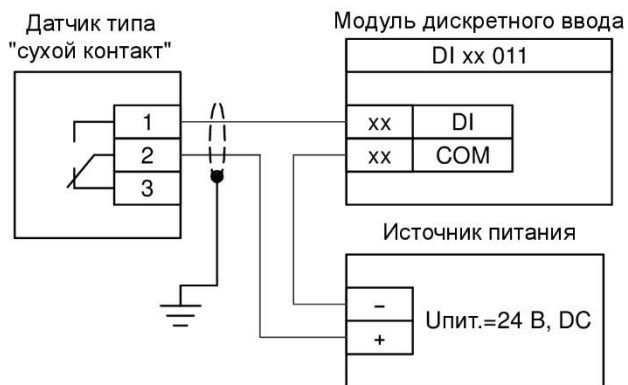
Рисунок Б.1.1 - Двухпроводная схема подключения датчика типа "сухой контакт" к модулям дискретного ввода
