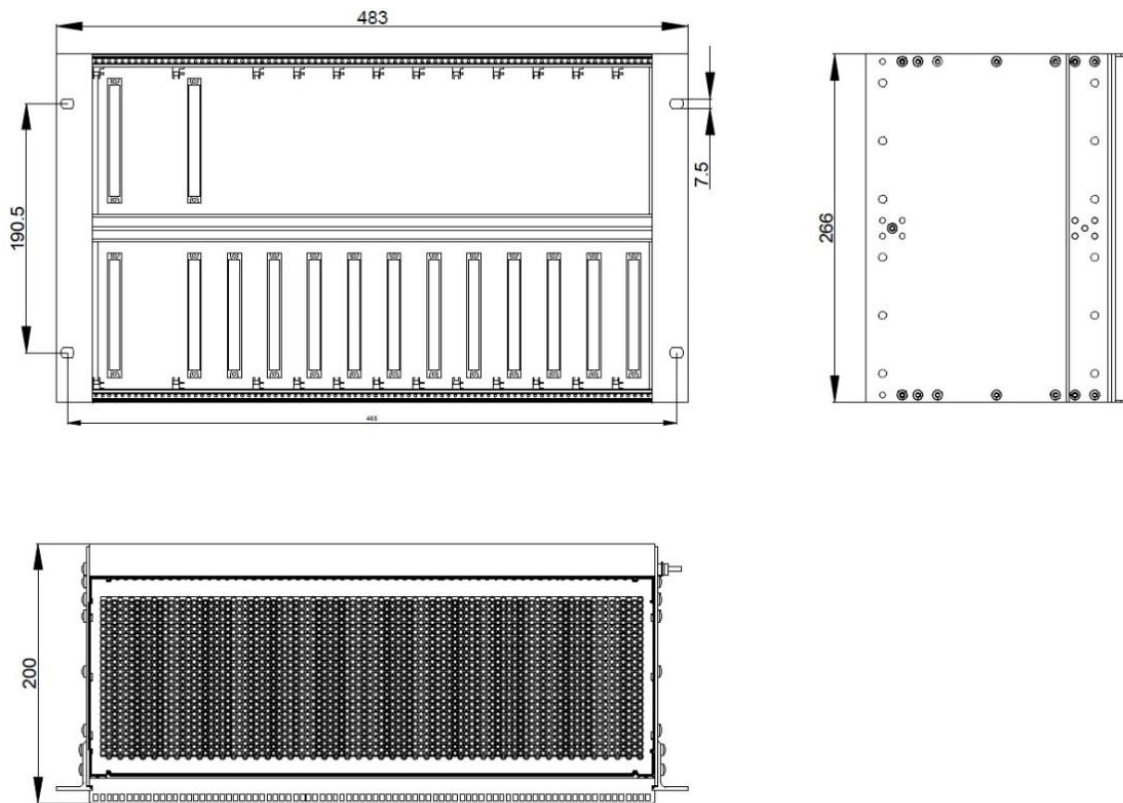
Рисунок 36 - Габаритные размеры крейга на 14 слотов (установка в 19" стойку)
