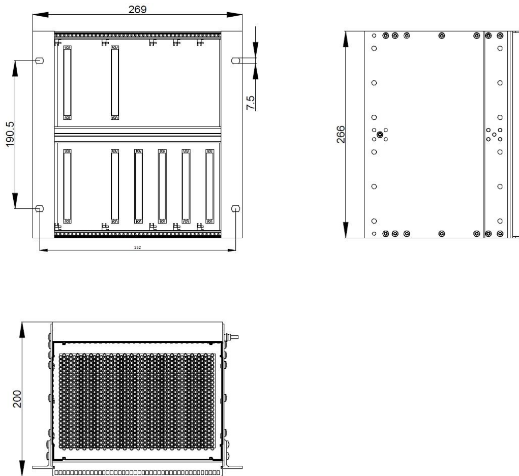
Рисунок 38 - Габаритные размеры крейта на 7 слотов (установка на 19" стойку)
