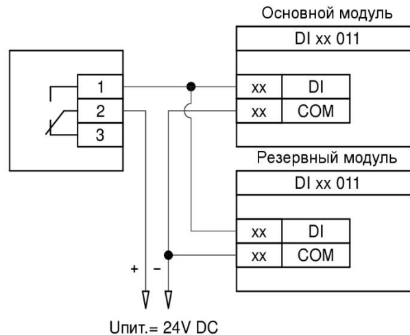
Рисунок В.1 - Подключение не резервированного датчика к резервированным каналам ввода дискретных сигналов
