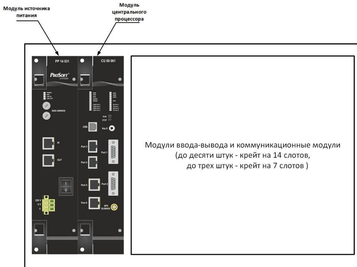
Рисунок 5 - Базовый крейт
