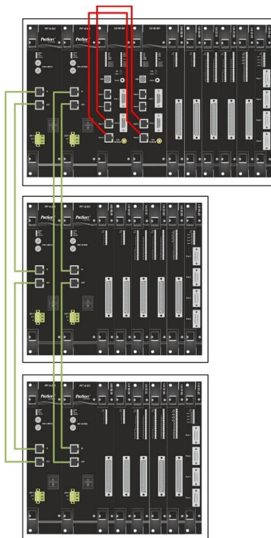
Рисунок 11 - Резервирование ЦП и БП
