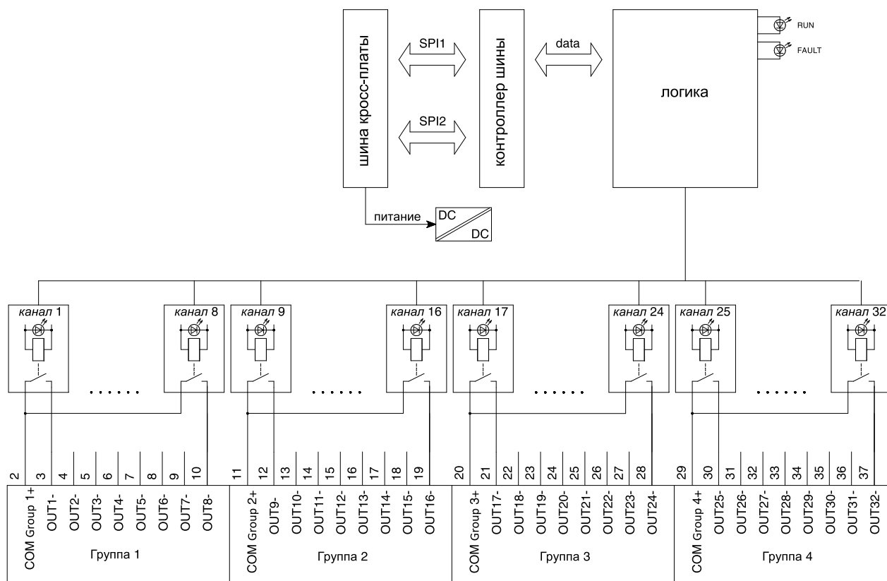
Рисунок 32 - Структурная схема модуля DO 32 011
