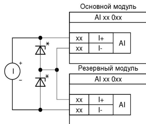
Рисунок В.3 - Подключение не резервированного датчика силы тока к резервированным каналам ввода аналоговых сигналов силы тока
