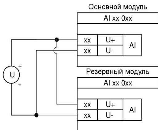
Рисунок В.2 - Подключение не резервированного датчика напряжения к резервированным каналам ввода аналоговых сигналов напряжения
