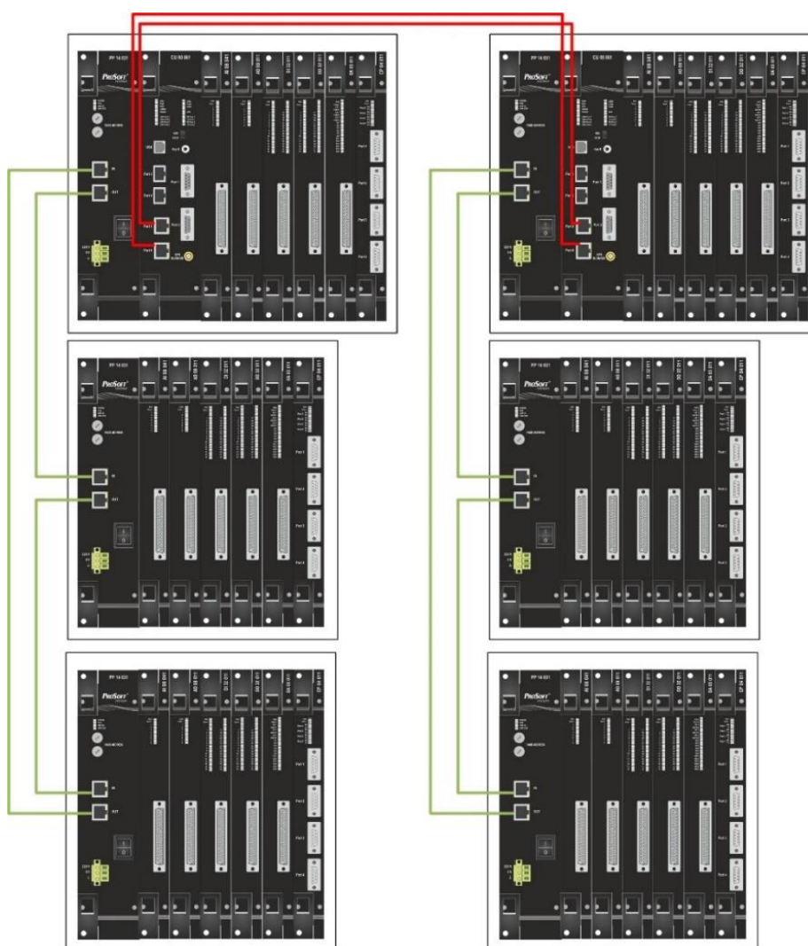
Рисунок 10 - Резервирование 100%
