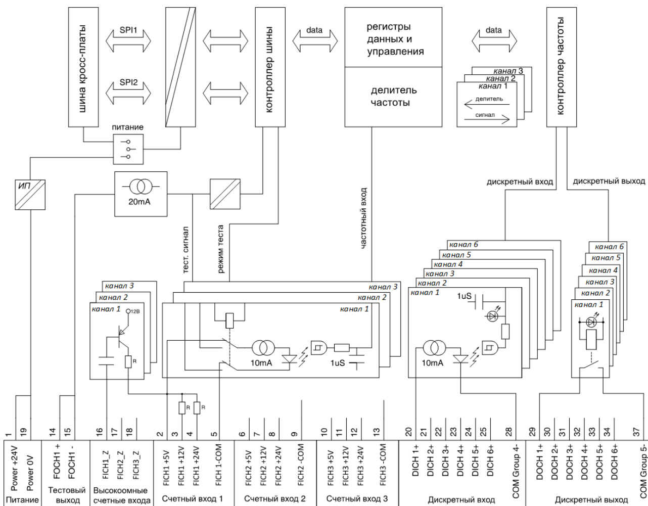
Рисунок 35 - Структурная схема модуля R600 DA 03 021
