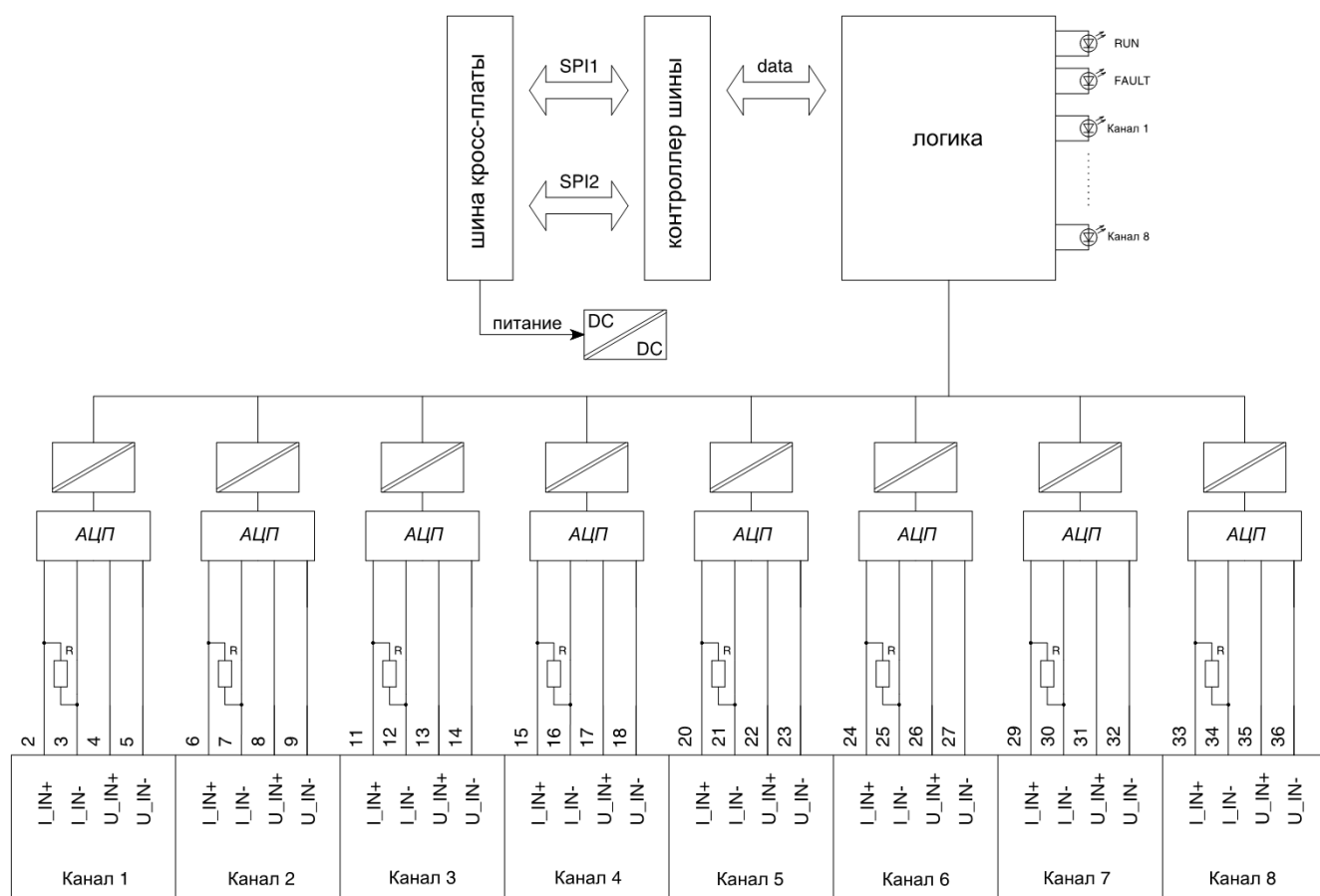
Рисунок 26 - Структурная схема модуля AI 08 041
