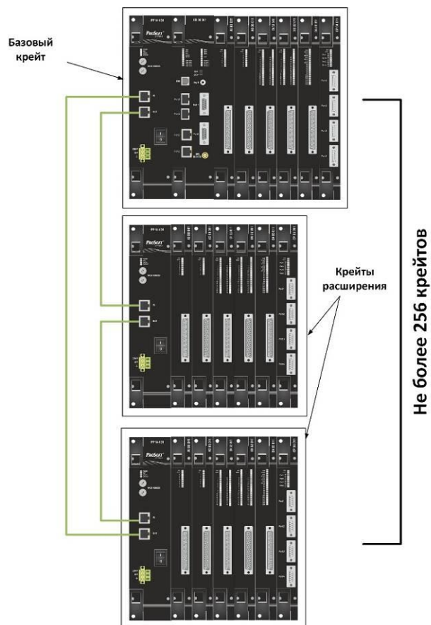
Рисунок 7 - Соединение кейтов по схеме «кольцо»
