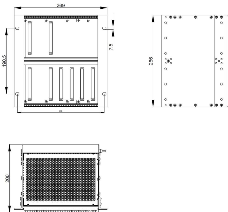
Рисунок 15 - Габаритные размеры крейта на 7 слотов при установке в стойку
